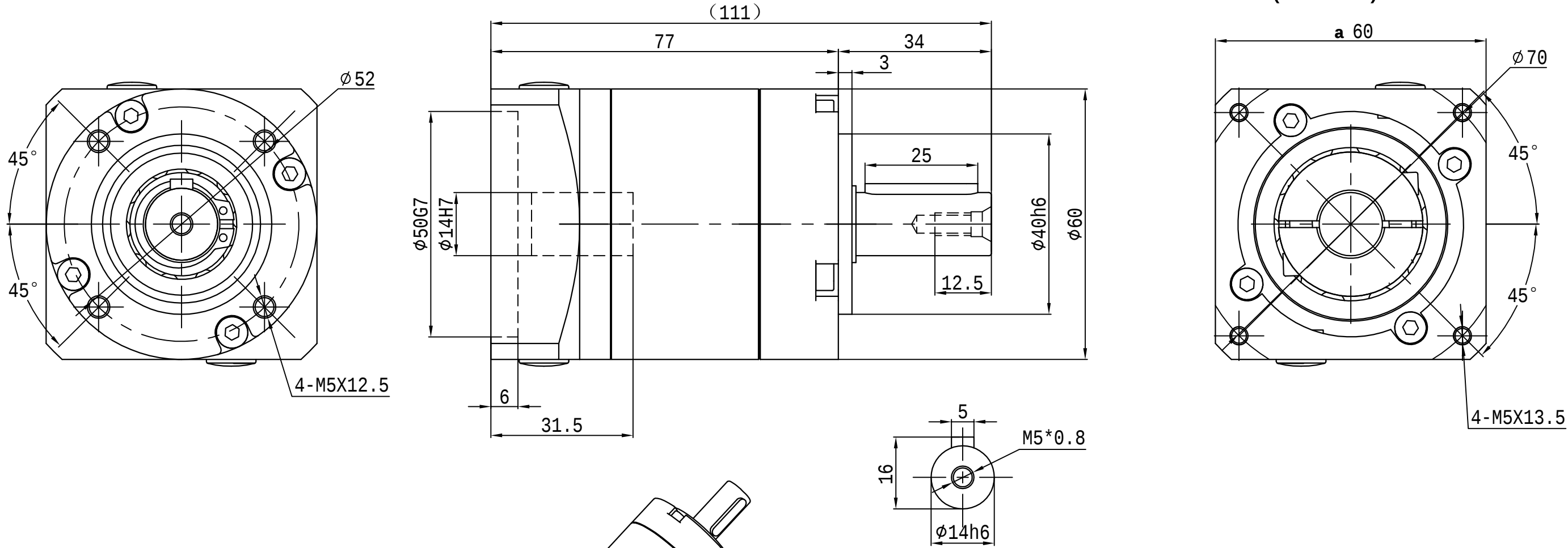
输出端 (OUTPUT)
