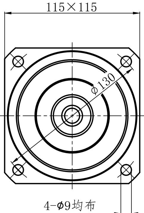
减速机输出端
