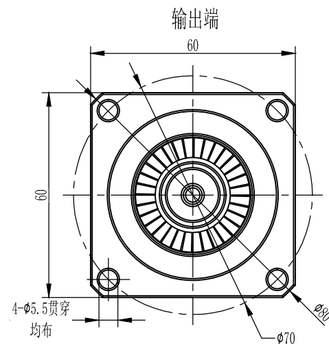
行星减速机技术参数 Technical parameters of planetary reducer
