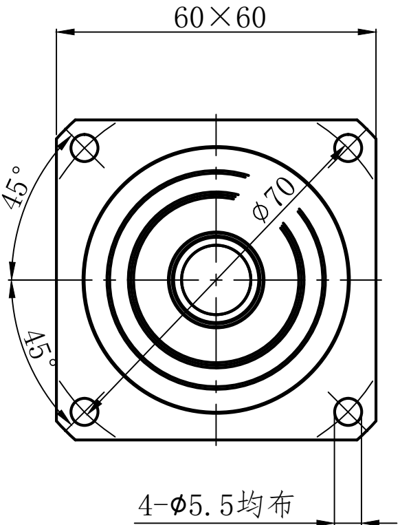
减速机输出端
