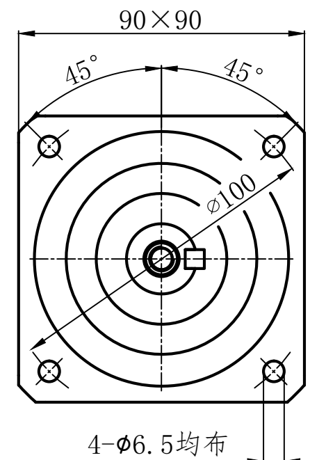
减速机输出端
