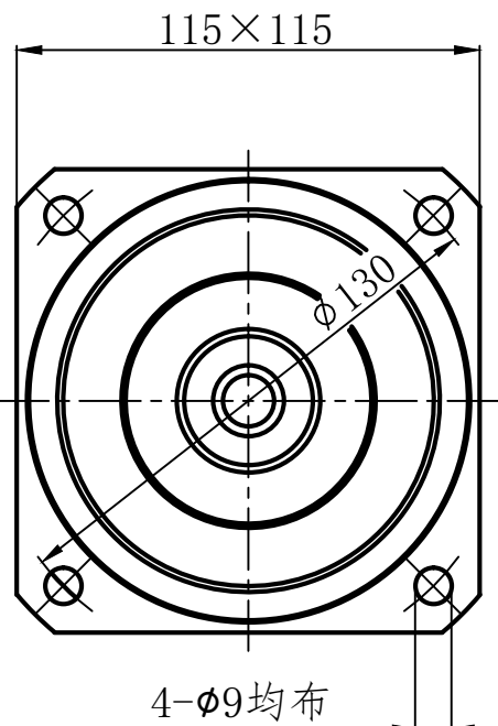
减速机输出端
