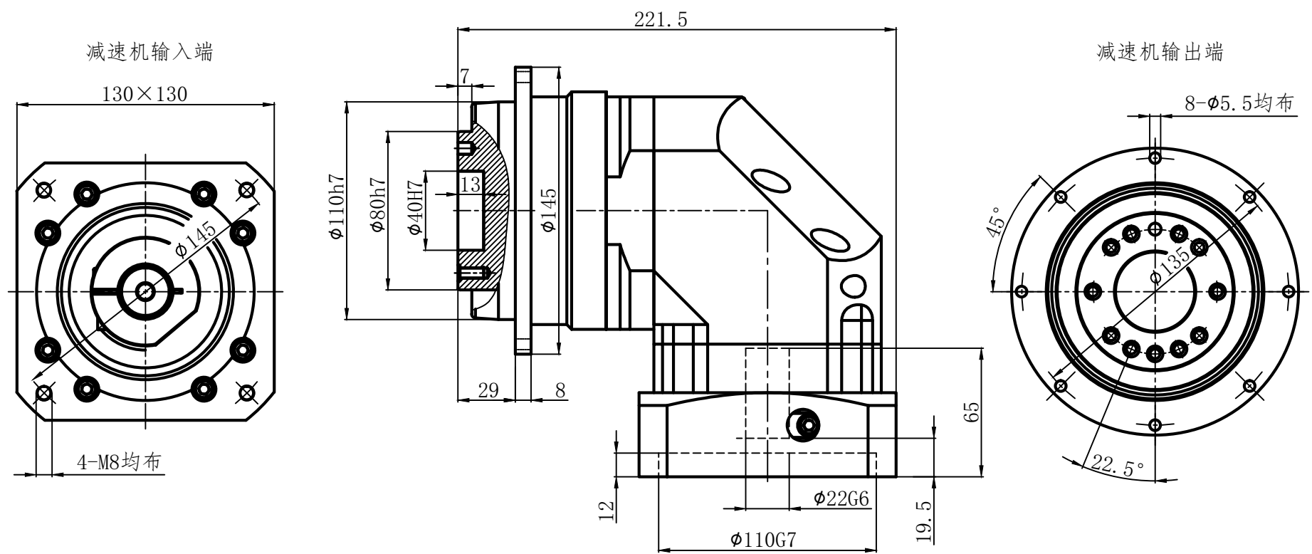
行星减速机技术参数 Technical parameters of planetary reducer
