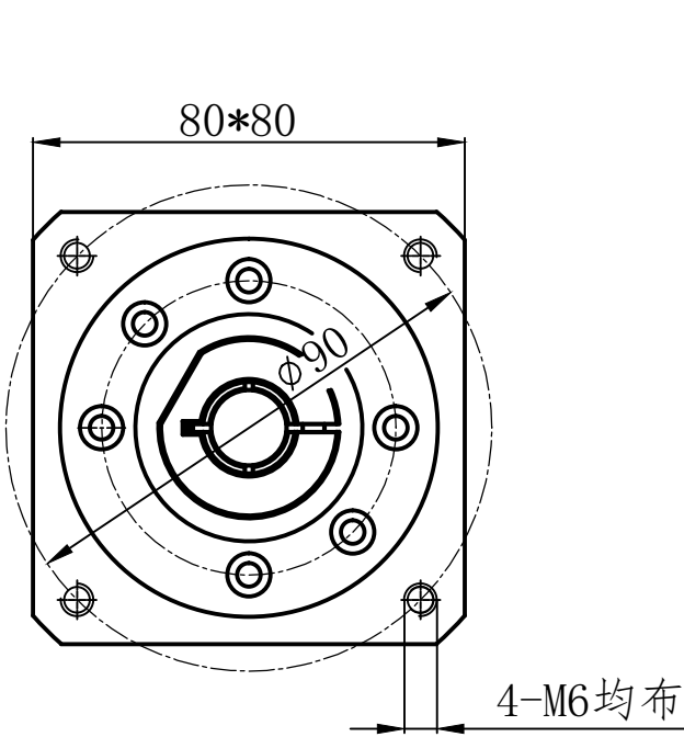
减速机输入端
