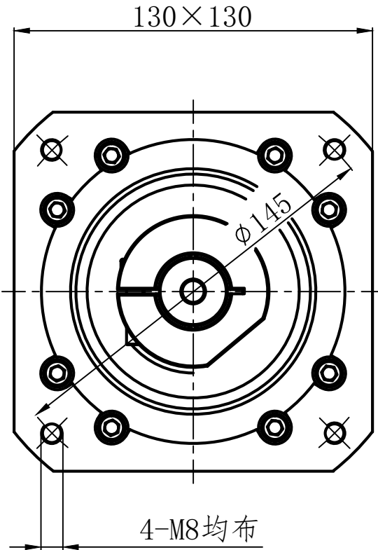
减速机输入端
