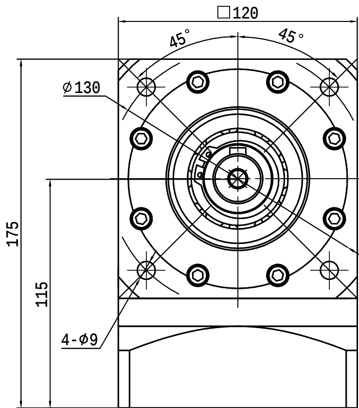
输出端 (OUTPUT)
