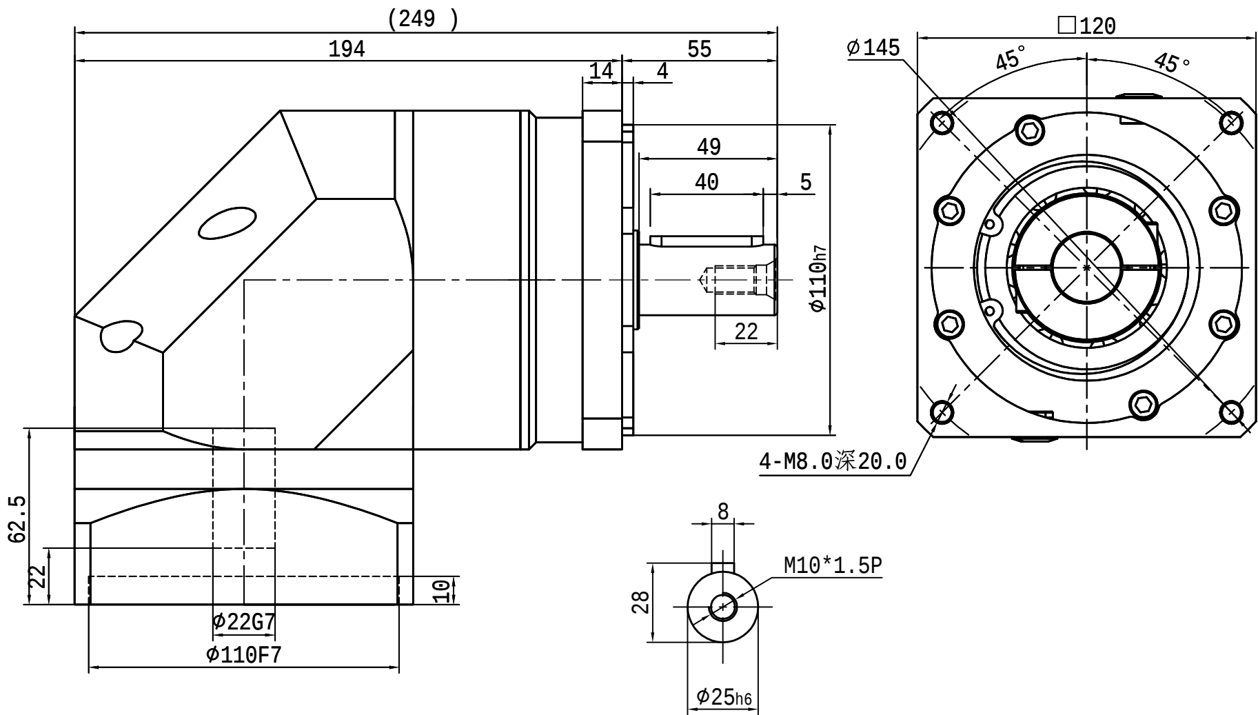
输入端 (INPUT)
